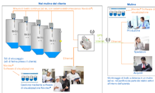
Esempio di gestione silo per i mulini e i loro clienti
